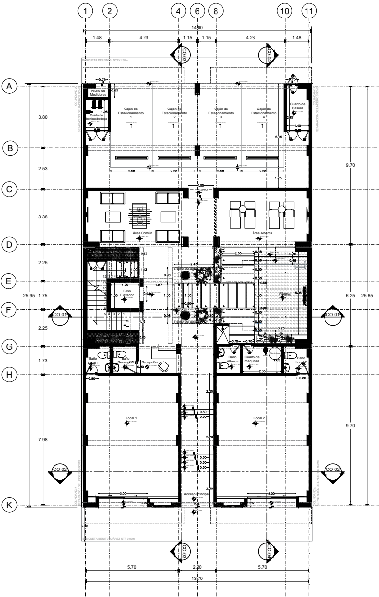
PLANTA ARQUITECTÓNICA
