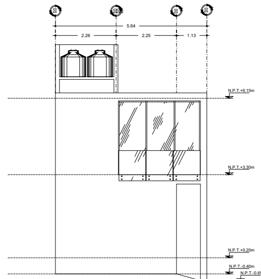
FACHADA POSTERIOR
